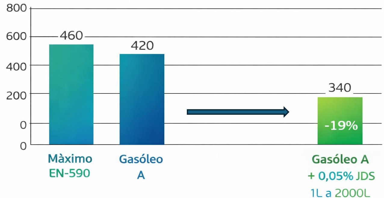
Test HFRR - Diésel (UNE ISO 12156-1)
